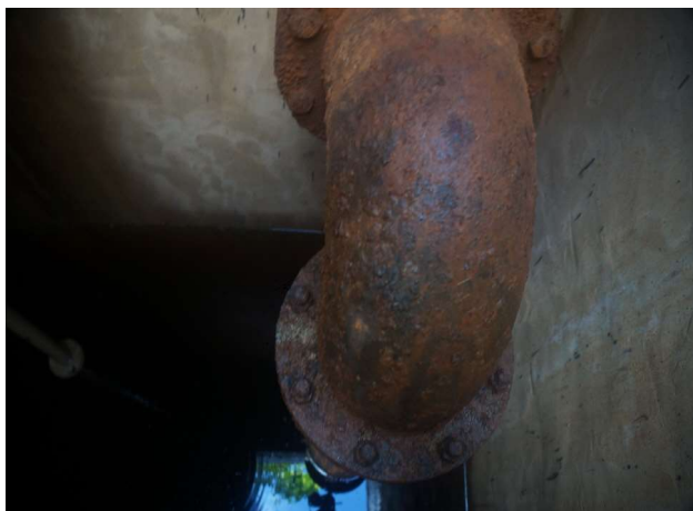
1지 유출밸브실 관부식
