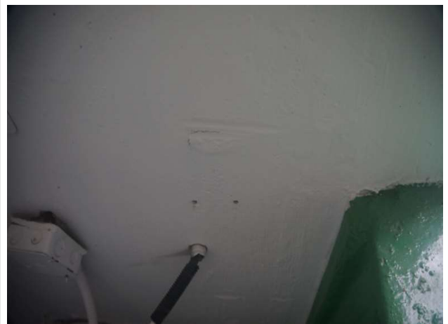
계단실 내부 벽체 들뜸(모르타르)
